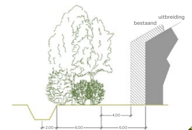
Figuur 8: Maatvoering erfsingels
